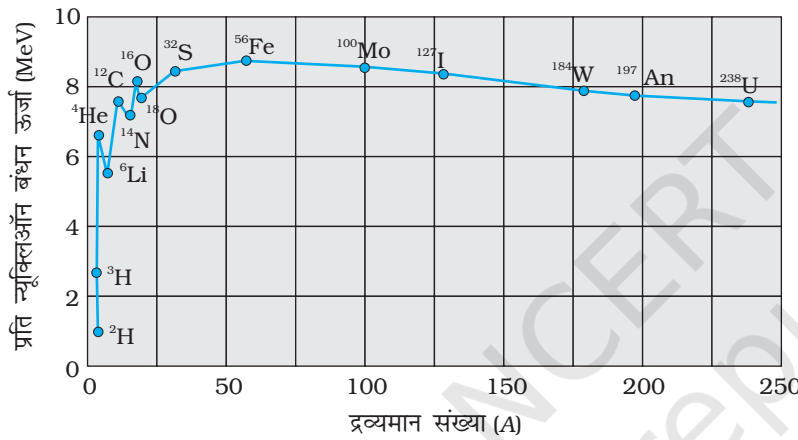
चित्र 13.1 द्रव्यमान संख्या के फलन के रूप में प्रति न्यूक्लिऑन बंधन-ऊर्जा।
