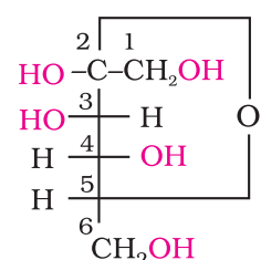
\beta - D - (-) - फ्रक्टोफ्यूरिनोस
