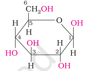
\beta - D - (+) - ग्लूकोपाइरैनोस
