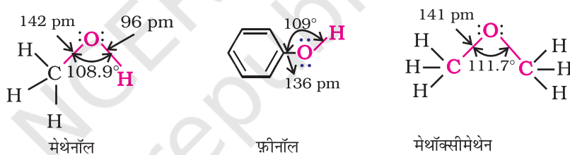
चित्र 11.1- मेथेनॉल, फ्रीनॉल तथा मेथॉक्सीमेथेन की संरचनाएँ
