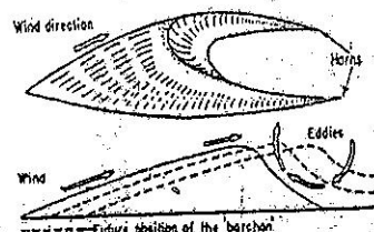
Fig. 2.9 Sand Dunes
