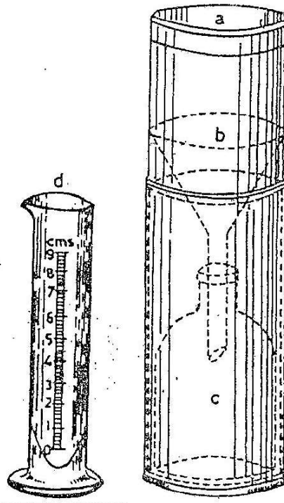
Fig. 4.5 Rain gauge
